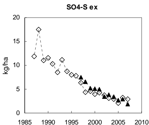
Figur 13. Svavelnedfall (exklusive havssaltsbidrag) till skogsmark i Knapanäs (◇) och Tagel (▲) (a) och nedfall av oorganiskt kväve (nitratkväve och ammoniumkväve) på öppet fält i Tagel (b) som årssumma på kalenderår (kg per hektar och år). De streckade linjerna i kvävefiguren visar gränserna för intervallet för kritisk belastning för kväve, 5-10 kg per hektar och år.
