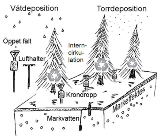
Figur 1. Principskiss för mätningarna. Nedfallet till skogsytorna består av vätdeposition och torrdeposition. Vissa ämnen interncirkuleras i trädkronorna vilket innebär att det som uppmäts i krondroppet är vätdeposition + torrdeposition ± interncirkulation.
