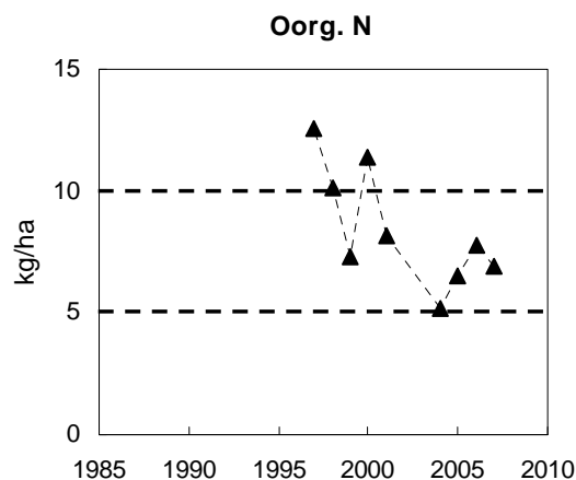
Figur 13. Svavelnedfall (exklusive havssaltsbidrag) till skogsmark i Knapanäs (◇) och Tagel (▲) (a) och nedfall av oorganiskt kväve (nitratkväve och ammoniumkväve) på öppet fält i Tagel (b) som årssumma på kalenderår (kg per hektar och år). De streckade linjerna i kvävefiguren visar gränserna för intervallet för kritisk belastning för kväve, 5-10 kg per hektar och år.
