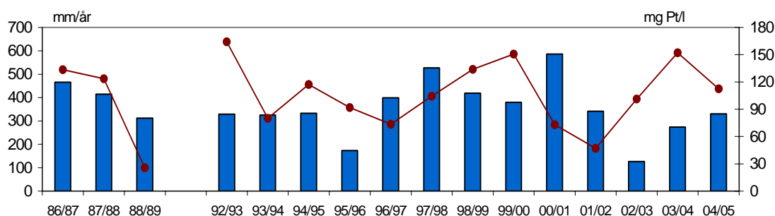
Figur 9: Årlig (hydrologiska år) avrinningsmängd (staplar, mm/år) och medelvattenfärg (heldragen linje, mg Pt/l) i bäcken vid Holmsvattnet.
