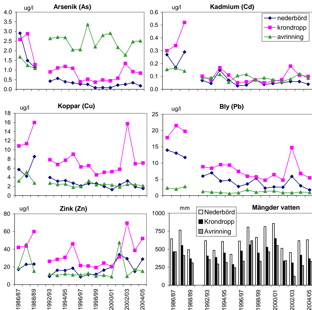
Figur 12: Volymvägda årsmedelvärden av halter i nederbörd på öppet fält och i kronddropp samt avrinning av arsenik och metaller vid Holmsvattnet (hydrologiska år).
