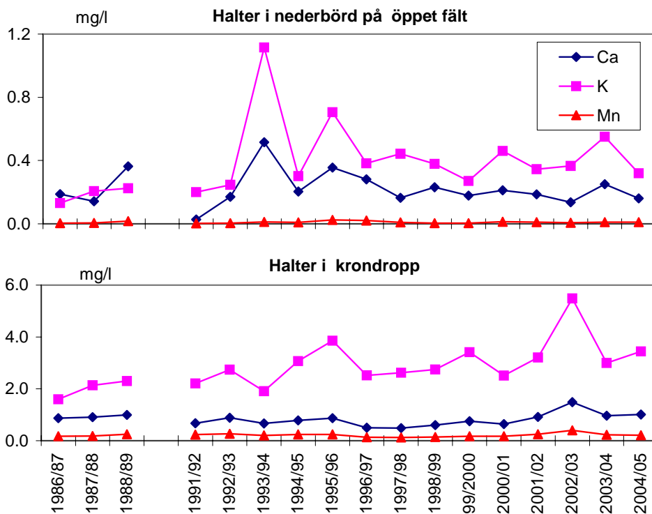
Figur 6: Volymvägda medelhalter av kalcium (Ca), kalium (K) och mangan (Mn) på öppet fält och i krondropp vid Holmsvattnet för hydrologiska åren 1986/87 till och med 2004/05. Notera att olika skalor används. Ett mätavbrott skedde under åren 1989-92.
