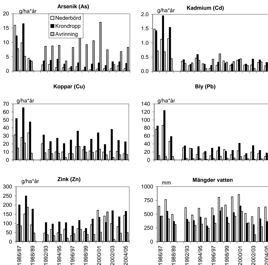
Figur 11: Metalltransporter (g/ha och hydr. år) i nederbörd, kronndropp och avrinning vid Holmsvattnet. Mängder vatten (mm/år) anges som referens.
