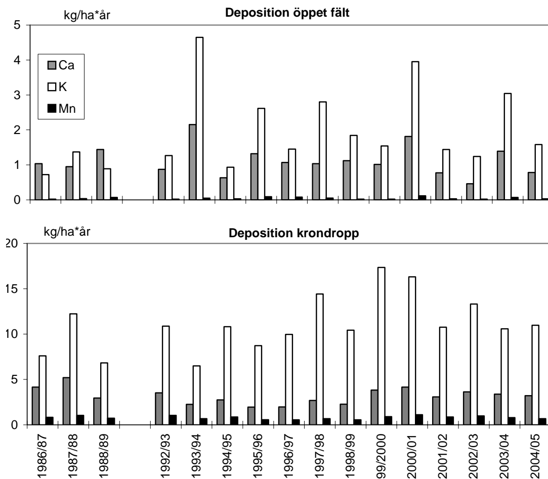
Figur 3: Deposition av i trädkronan interncirkulerande ämnen kalcium (Ca), kalium (K) och mangan (Mn) på öppet fält och i krondropp vid Holmsvattnet för hydrologiska åren 1986/87 till och med 2004/05. Notera att olika skalor används. Ett mätavbrott skedde under åren 1989-92.
