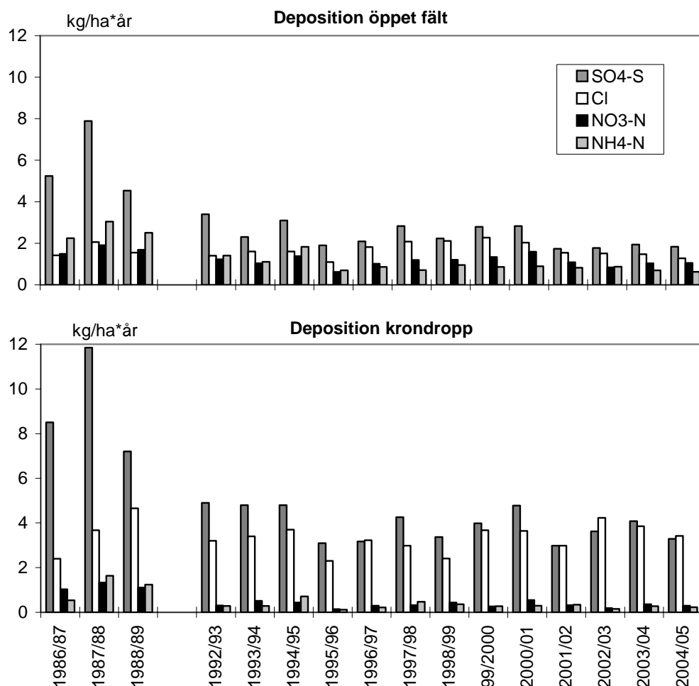
Figur 2: Deposition av svavel, klorid och kvävekomponenter på öppet fält och i kronddropp vid Holmsvattnet för hydrologiska åren 1986/87 till och med 2004/05. Ett mätavbrott skedde under åren 1989-92.
