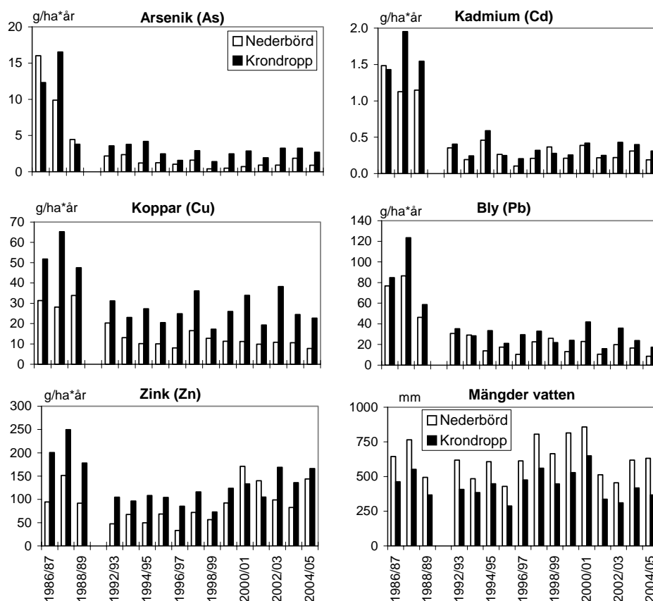
Figur 4: Deposition av arsenik och metallerna kadmium (Cd), koppar (Cu), bly (Pb) och zink (Zn) vid Holmsvattnet mellan oktober 1986 och september 2005. Ett mätavbrott skedde åren 1989-92.
