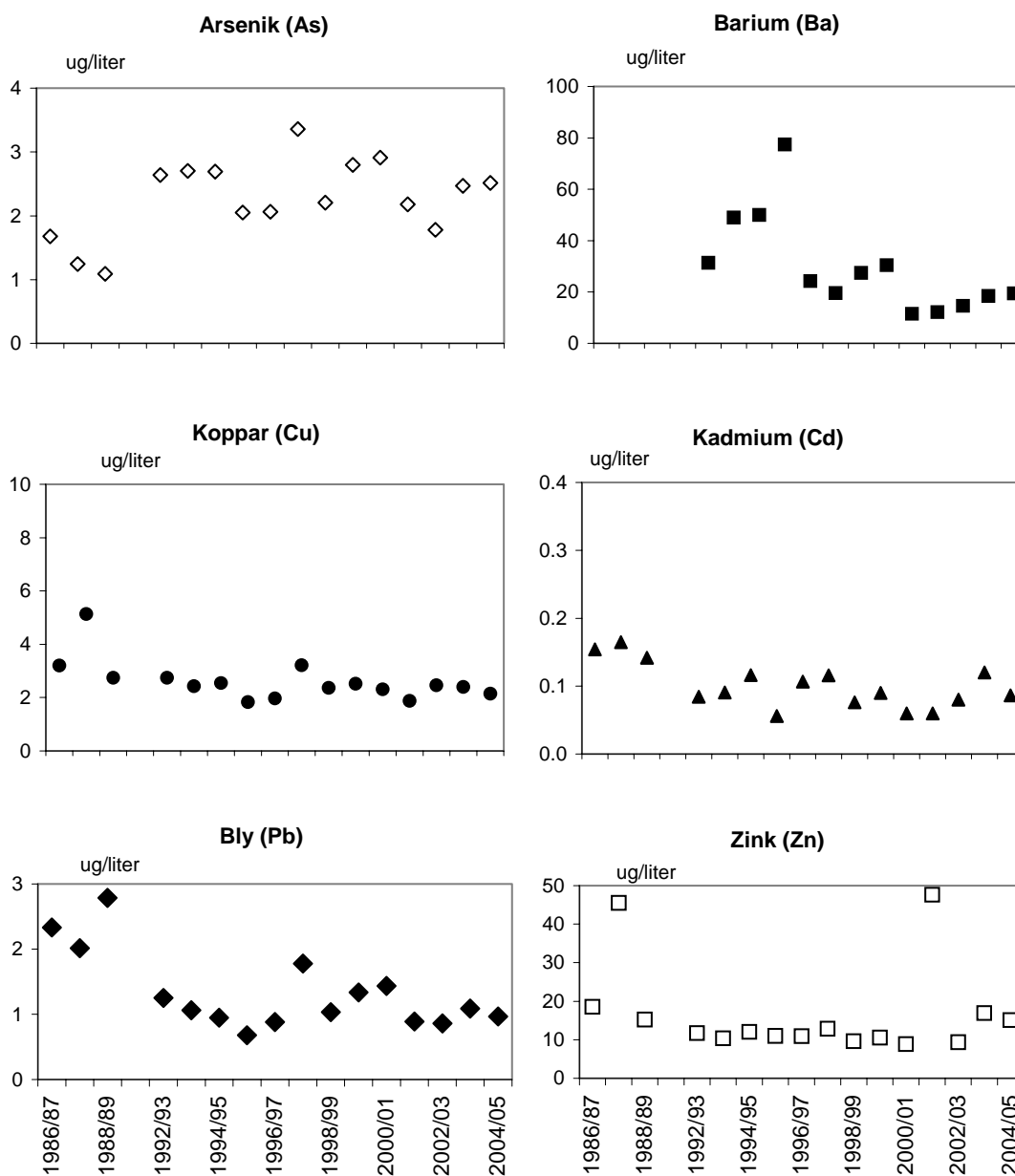
Figur 10: Volymvägda årsmedelvärden av halter av arsenik och metaller i avrinning från Holmsvattenområdet nära Rönnskärsverken för hydrologiska åren 1986/87 t o m 2004/05.
