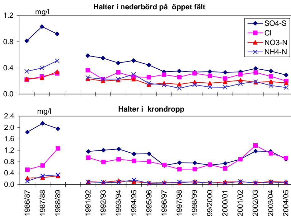
Figur 5: Volymvägda medelhalter av svavel, klorid och kvävekomponenter på öppet fält och i krondropp vid Holmsvattnet för hydrologiska åren 1986/87 till och med 2004/05. Notera att olika skalor används. Ett mätavbrott skedde under åren 1989-92.
