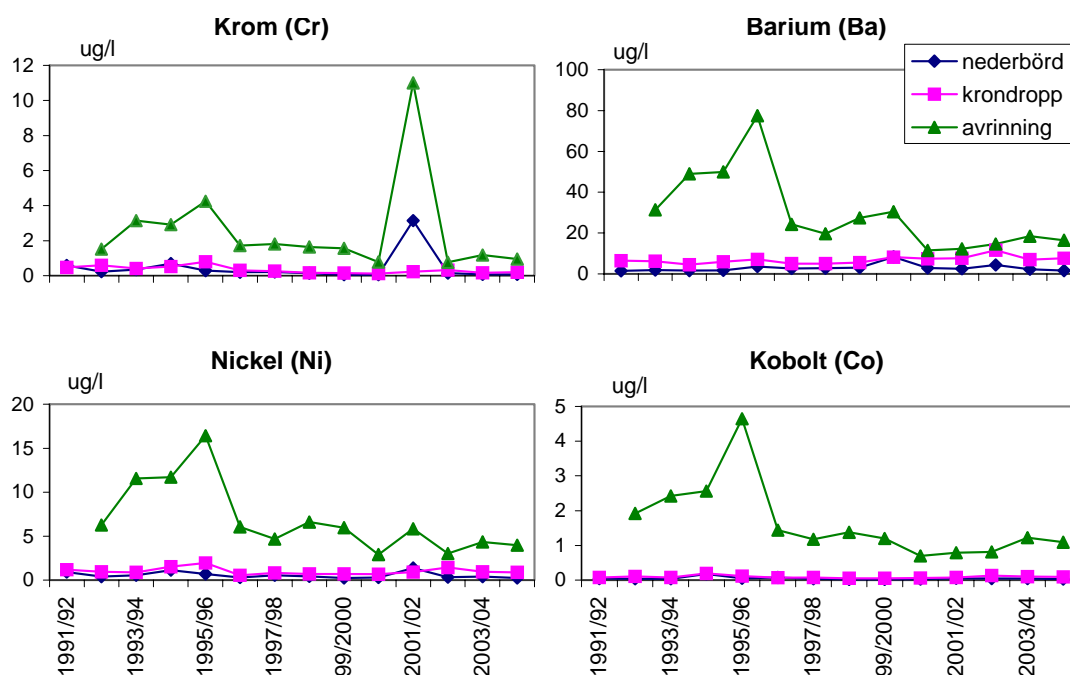
Figur 13: Haltvariationer (hydrologiska årsmedelvärden) av krom, barium, nickel och kobolt i nederbörd, kronddropp och avrinning från Holmsvattenområdet.
