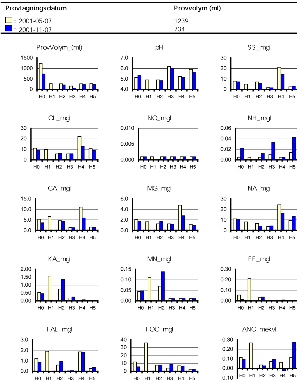
Figur 6. Markvattendata från två provtagningar i Rockneby. H1-5 är analysresultat av delprov från lysimeter 1-5. H0 är beräknat volymvägt värde för generalprov från dessa delprov.
