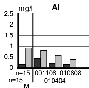
Figur 13. Depositions- och markvattendata från Humlered, P 93.
