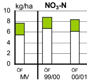
Figur 10. Depositionsdata (öppet fält) från Lurås, P 90.
