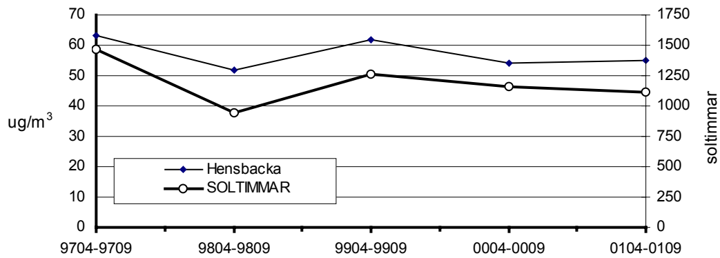
Figur 19. Somarmedelvärden (april-september) för marknära ozon ( O_3 ) i Hensbacka under 1997-2001 samt antal soltimmar under samma period i Göteborg.
