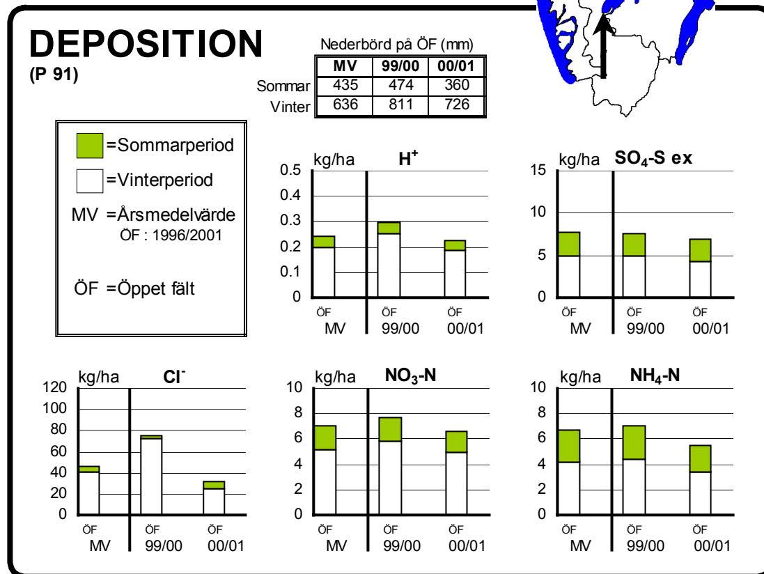
Figur 11. Depositionsdata (öppet fält) från Lindås, P 91.
