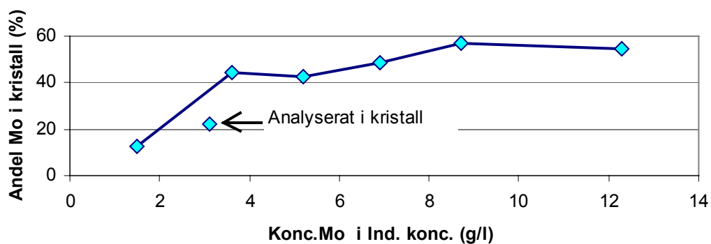
Figur 2.3 Kristallisationsgraden för Mo avsatt mot koncentrationen Mo i industningskoncentratet. Kristallisationsgraden för Mo är beräknad genom differensen mellan mängden Mo i ursprunglig syra före industning/kristallisation och mängden Mo i moderluten (filtratet) som erhålls efter kristallisation. Gäller ej för punkten ”Analyserat i kristall”.
