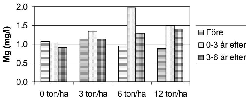
Figur 9d. Magnesiumhalt i markvattnet före och efter behandling med finmald dolomit (medelvärden från samtliga mätningar).
