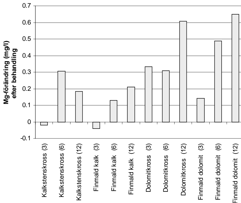
Figur 8. Förändring av magnesiumhalt i markvattnet efter behandling i förhållande till förändringen i referensytorna. Förändringen avser perioden före behandling jämfört med perioden 3-6.5 år efter behandling.
